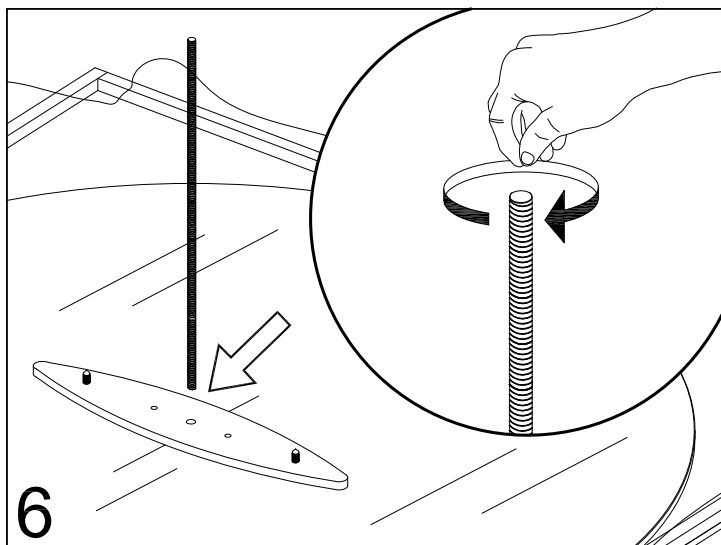
6 Avvitare manualmente la barra filettata alla piastra del cristallo. Fasten the threaded rod properly with hand to the glass board.
