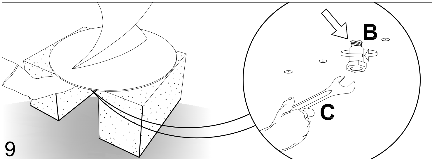
9 Per stringere il piano in cristallo alla base, infilare la mano sotto la piastra in metallo e con la chiave in dotazione avvitare il bullone (B). Sollevare delicatamente il tavolo in due persone e appoggiarlo con cura a pavimento.
