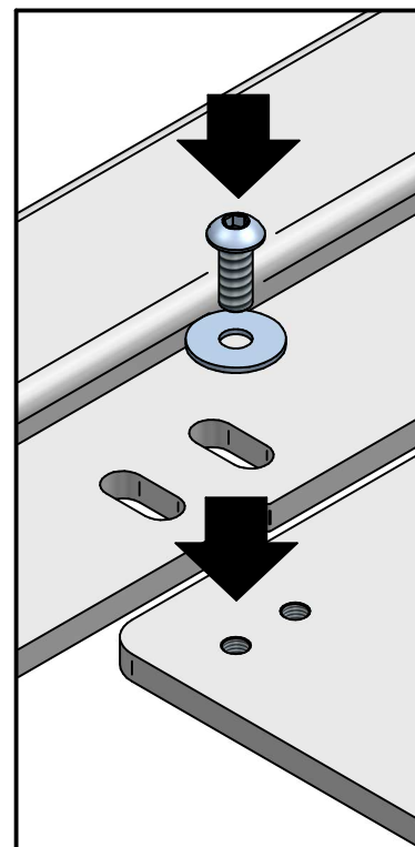
n° 08 rondella ø8x24 N.
