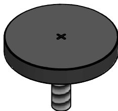
N°2 Ø60 M10x35 Ne
